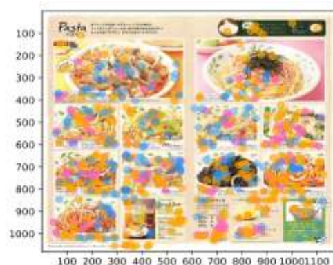
▲感性マップ
